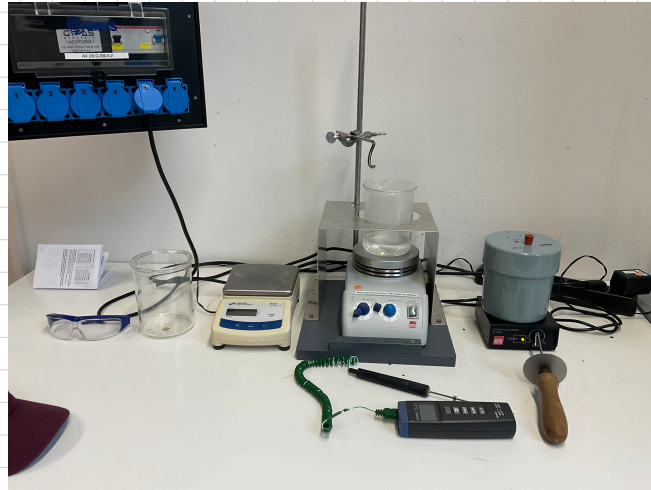
Abb. 3.1: Messaufbau
